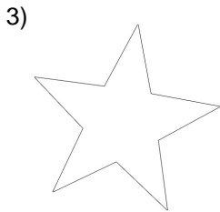
star
